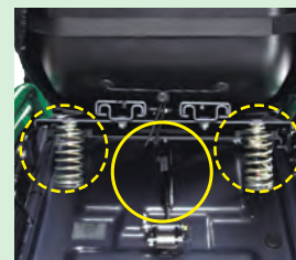
シート下のスプリングとガスダンパーで クッション性向上
